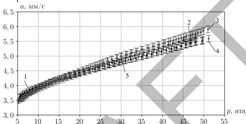
Рис. 1. Зависимости скорости горения от давления:
