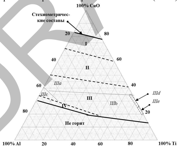
Рис.1. Режимы горения смесей оксида меди с алюминием и титаном.
