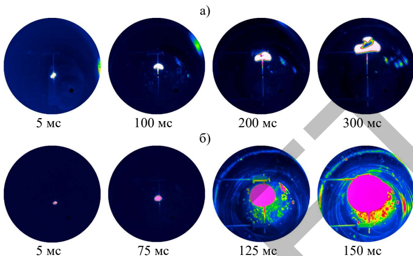
Рисунок 1 – Кадры распространения пламени в эксперименте вблизи: а) НКПВ и б) ВКПВ. Диаметр кадров – 150 мм.
