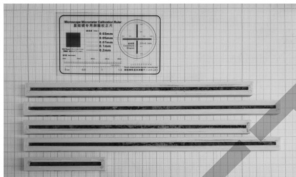
Рис. 1. Внешний вид образцов, содержащих энергоемкую смесь ПК — перхлорат бария
