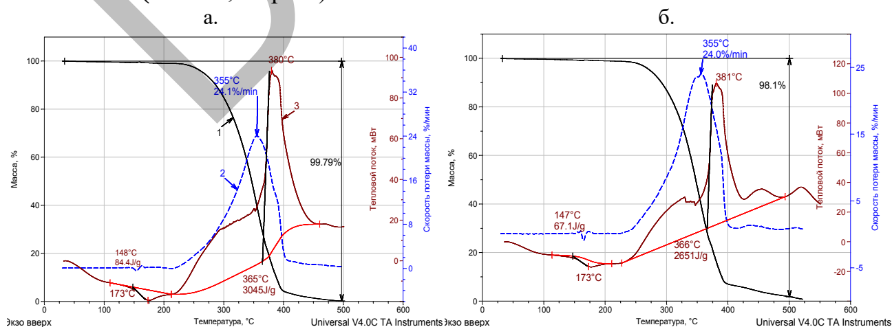
Рисунок 2. ТГ (1), ДТГ (2) и ДСК(3) кривые образца ковровой дорожки Bal Tekstil Karavan W490A, (а) и образца ковровой дорожки ОВАМ Yke, (б) (20 °С/мин; атмосфера – воздух).
