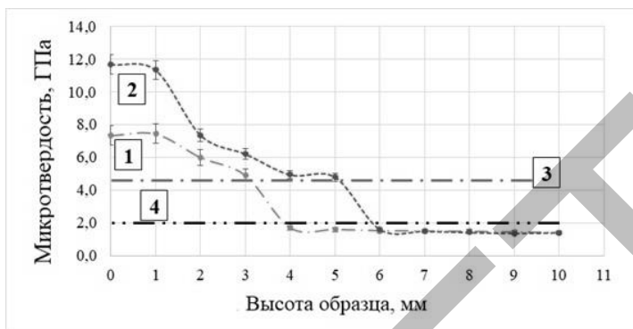
Рис.1. Микротвёрдость наплавочных покрытий и исходной подложки: 1 – 180 А, 2 – 200 А, 3 – сталь 65Г после ТО, 4 – сталь Ст3
