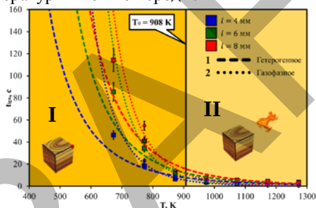
Рис. 1. Зависимости времён задержки зажигания (1 – гетерогенного и 2 – газофазного) от температуры окислителя пространства для древесины: сосны I – область гетерогенного зажигания, II – область газофазного зажигания.
