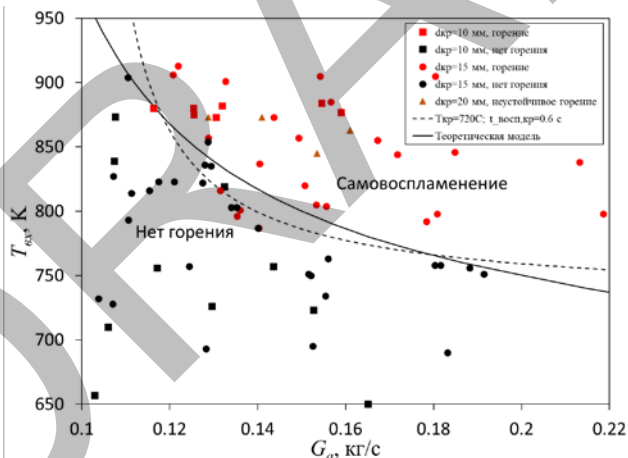
Рис. 2 – Граница самовоспламенения, построенная по экспериментальным данным (обозначен пунктирной линией) и с помощью теоретической модели (сплошная линия).
