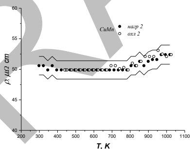
Рис. 1 – Зависимость удельного электросопротивления от температуры сплава на основе системы Cu-Mn
