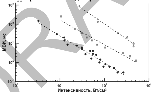
Рисунок 1 Зависимости минимального воспламеняющего импульса от интенсивности излучения. ●- 405 нм; ■-520 нм; ◆- 785 нм.
