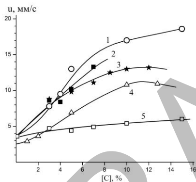
Рис.2. Зависимости скоростей горения композиций на основе ПХА от концентрации: ПГБ №3 (1); ПГБ №4 (2); ферроцена (3); изопренового каучука СКИ-3 (4) и \text{Al}_2\text{O}_3 (5).
