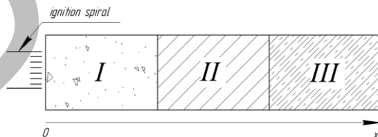
Рис.1 Схема трехслойной системы. I – Ti-C; II – Углеродистая сталь; III – Ni-Al
