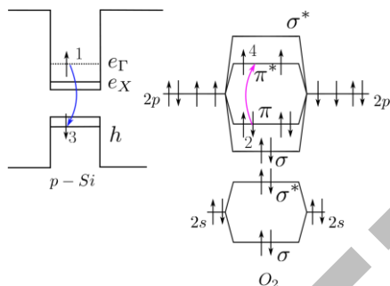
Рис.1. Механизм резонансной передачи энергии от кремния к молекуле кислорода с образованием радикала кислорода. На рисунке слева показана зонная диаграмма p-Si как квантовая яма.
