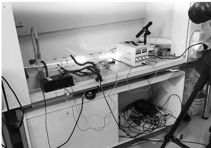
Рис. 1. Протекание экзотермической реакции ПК и перхлората бария в контейнере диаметром 0.7 мм и длиной 15 см.
