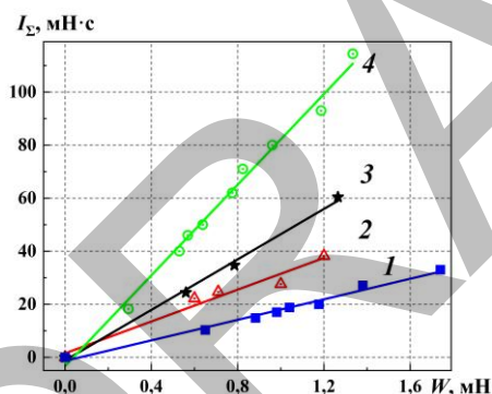
Рис. 1. Импульс тяги ( I_{\Sigma} ) микротрастера с соплом в зависимости от веса топлива ( W ):
