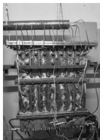
Рисунок (б) — Фотография экспериментального стенда
