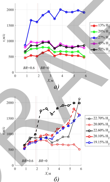
Рисунок 1 – Зависимость оценочной скорости фронта пламени
