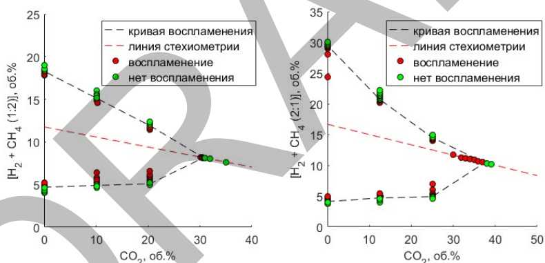
Рисунок 2 – Пределы воспламенения смеси \text{H}_2\text{-CH}_4\text{-воздух-CO}_2
