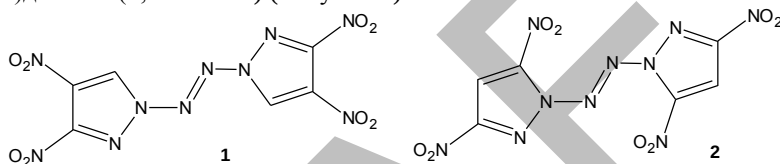
Рисунок 1. Структурные формулы изученных соединений: 1 - 3,4-DNPAz; 2 - 3,5-DNPAz
